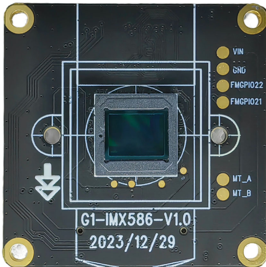
Vorderansicht
